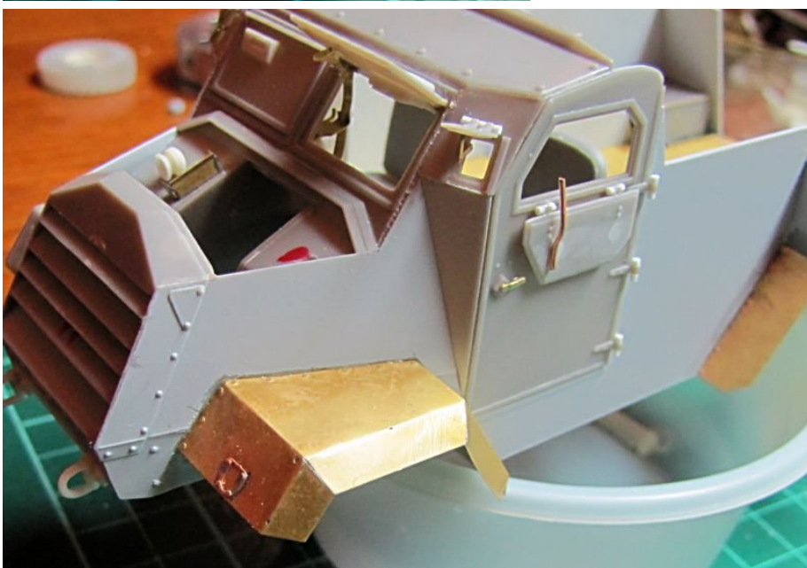
PE A and PE B front and rear mudguards
